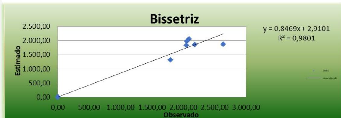
Gráfico – Bissetriz dos quadrantes ímpares.
